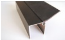
Üst Sızdırmazlık Fitali
